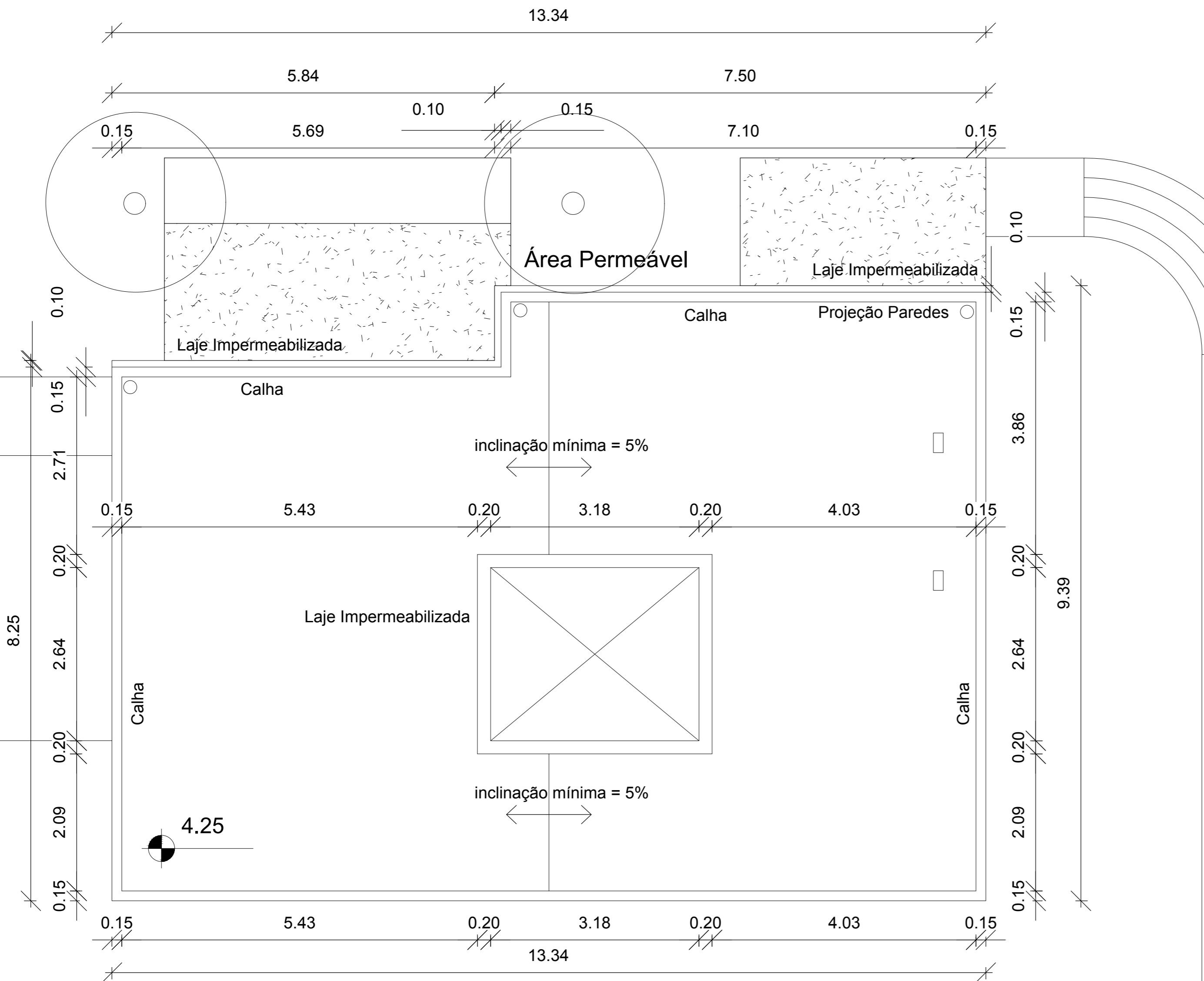
PLANTA DE COBERTURA ESC 1/50
